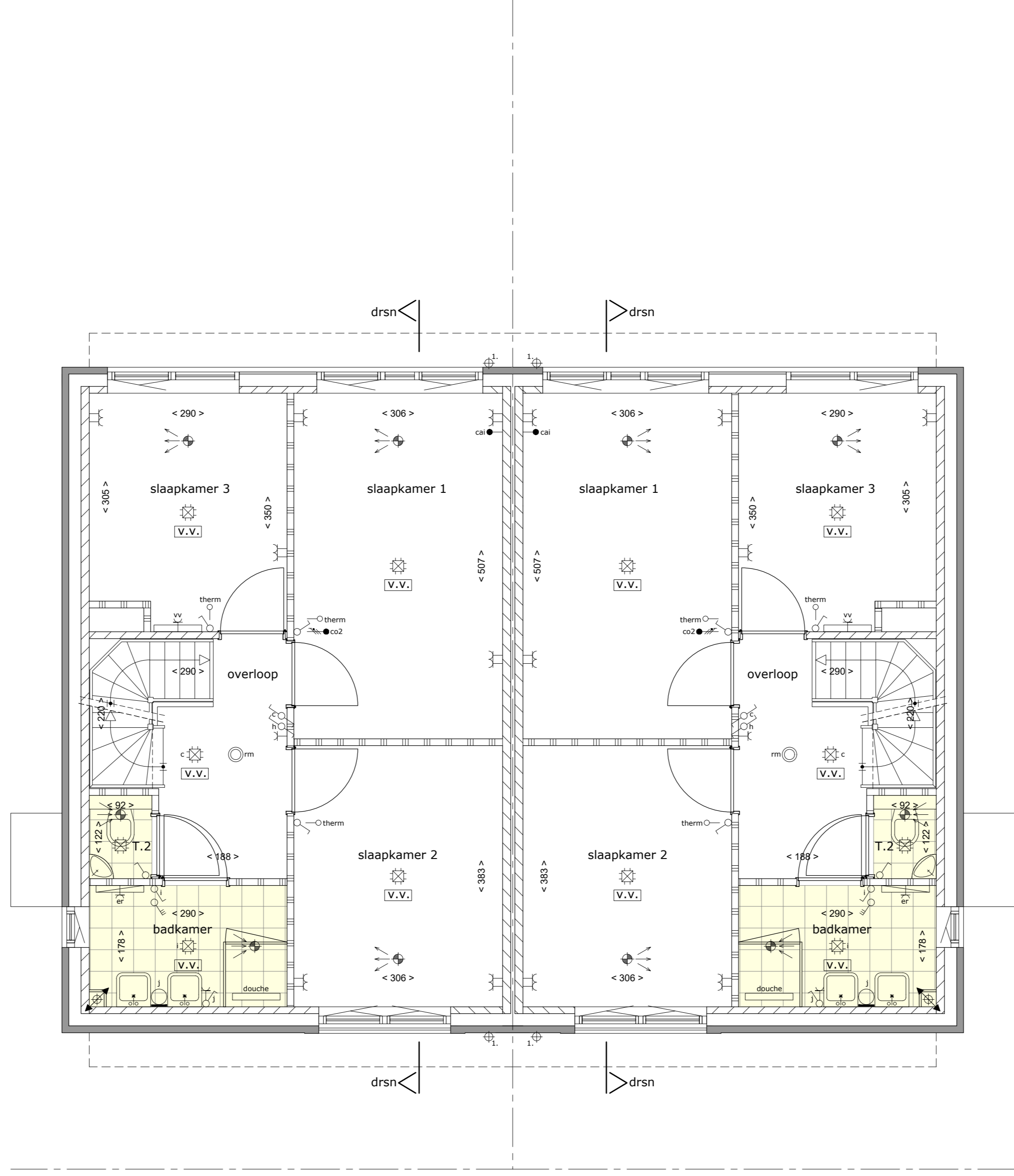
kavel 107 kavel 108 1ste verdieping schaal 1:50
