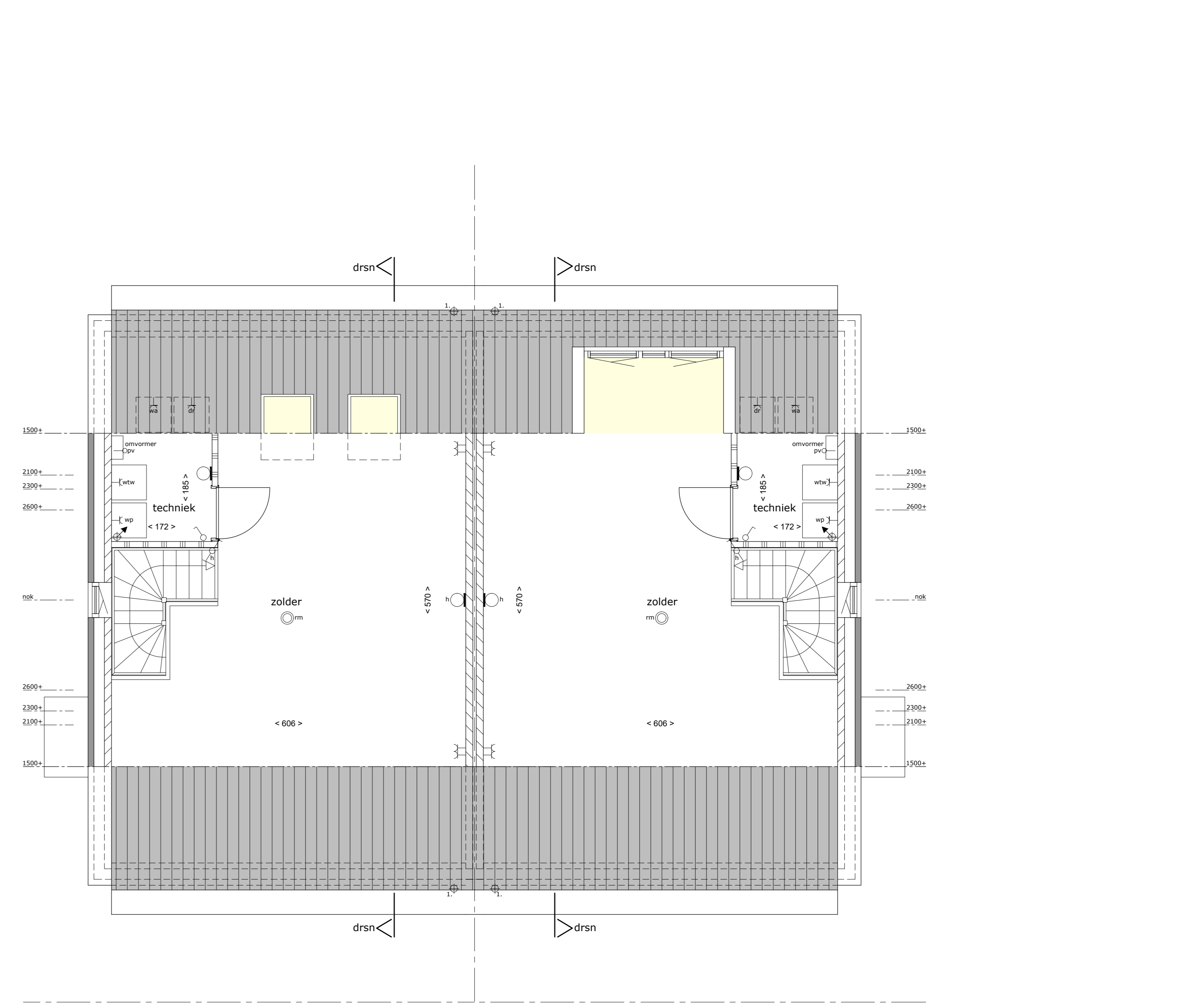
kavel 107 kavel 108 2de verdieping schaal 1:50
