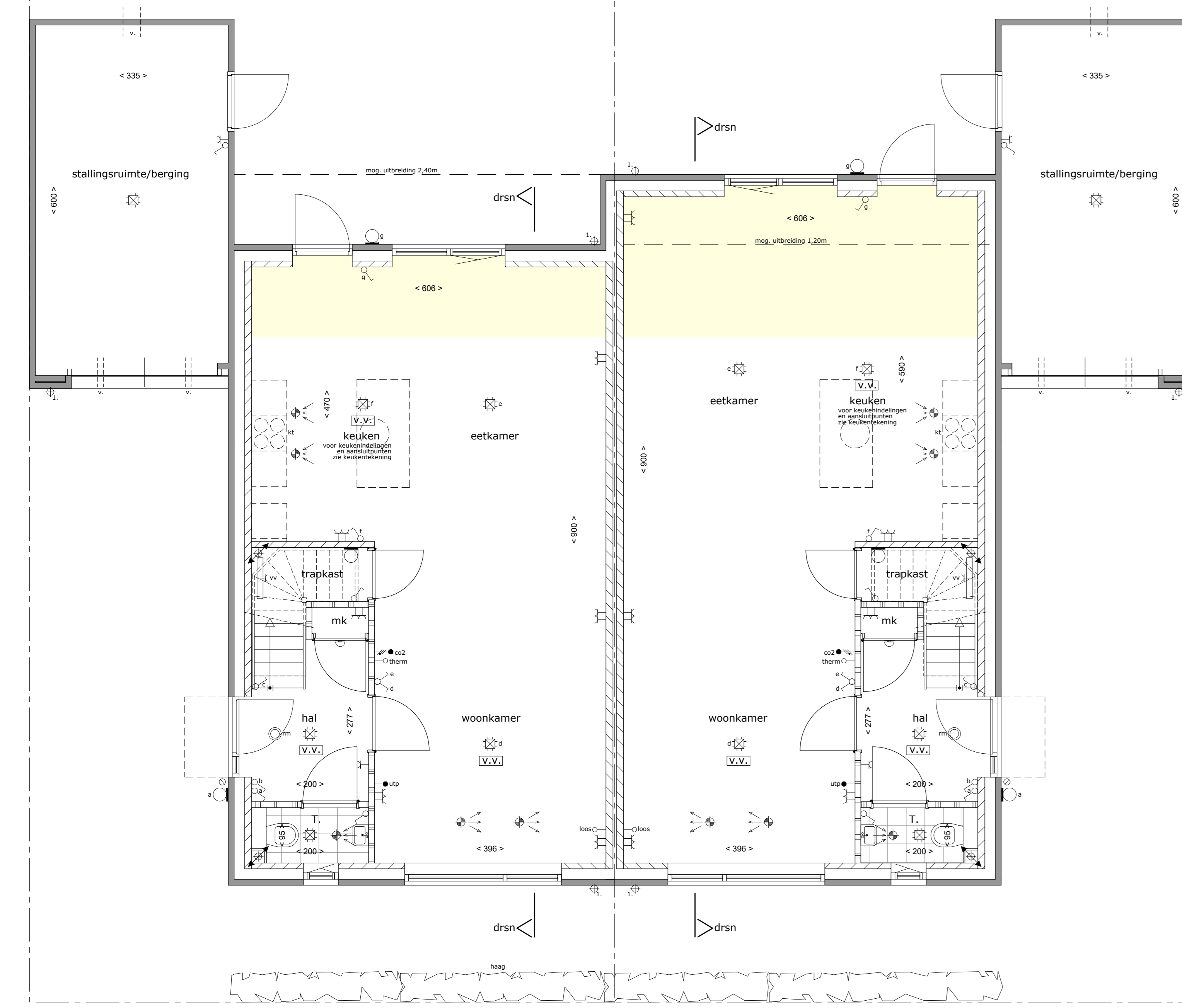
kavel 107 kavel 108 begane grond schaal 1:50
