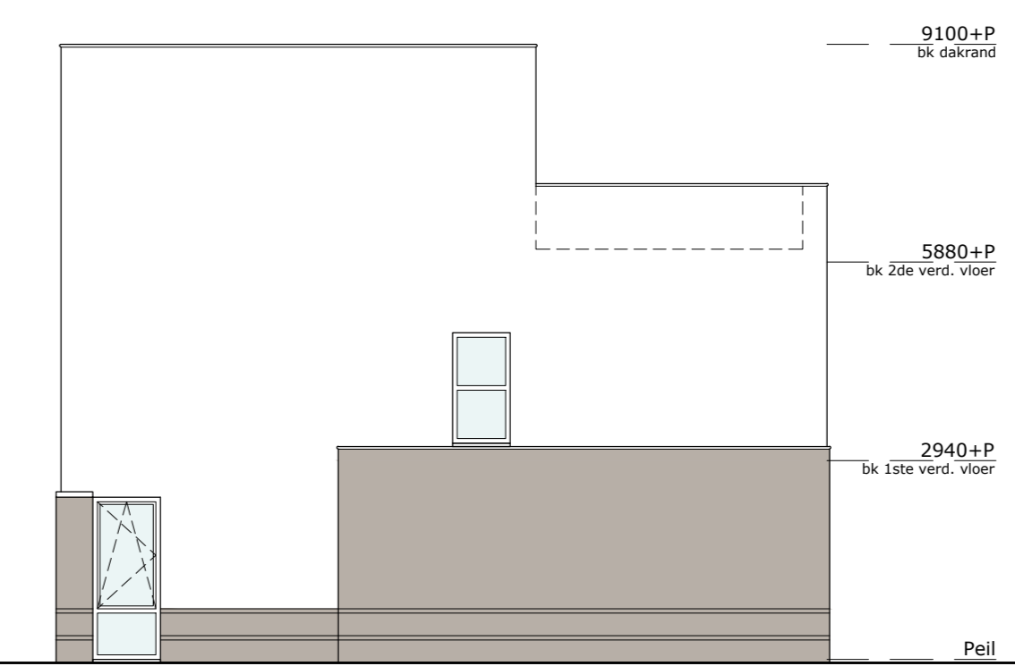
rechterzijgevel schaal 1:100 OPTIE: VERGROTEN HOBBYRUIMTE
