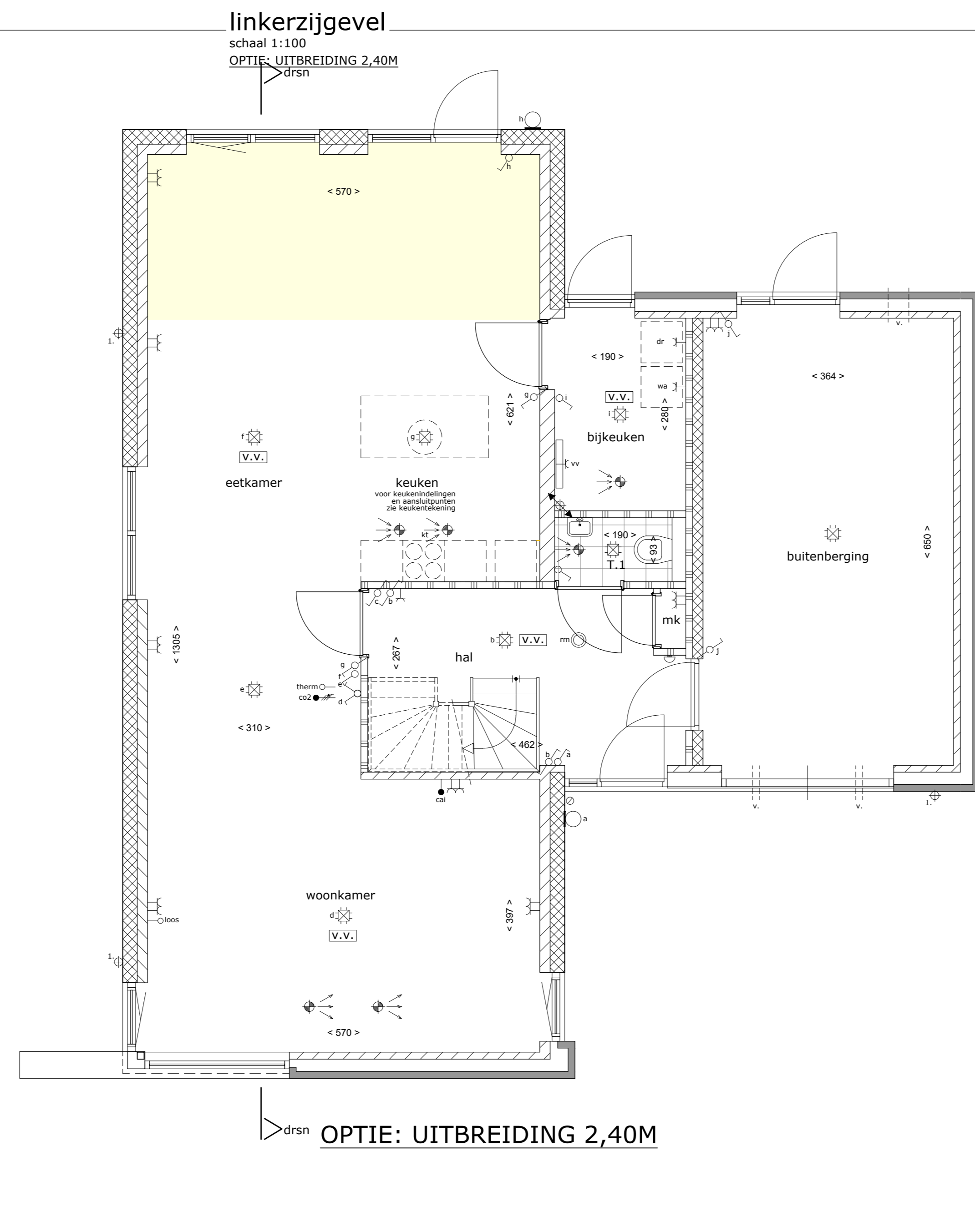
begane grond schaal 1:50
