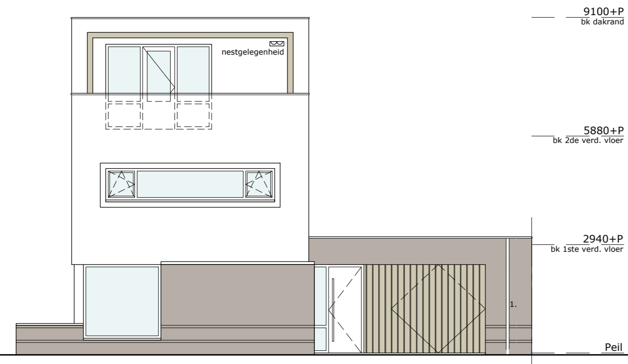
voorgevel schaal 1:100 OPTIE: UITBREIDING 2,40M
