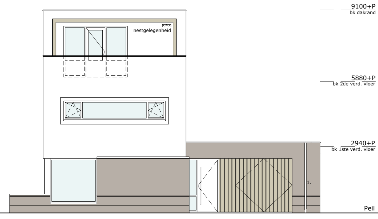
voorgevel schaal 1:100 OPTIE: UITBREIDING 1,20M
