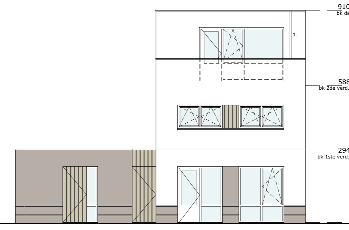
achtergevel schaal 1:100 OPTIE: UITBREIDING 1,20M
