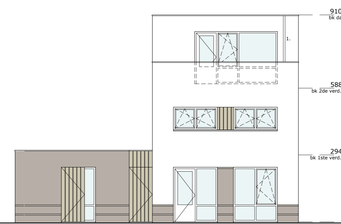
achtergevel schaal 1:100 OPTIE: VERGROTEN HOBBYRUIMTE
