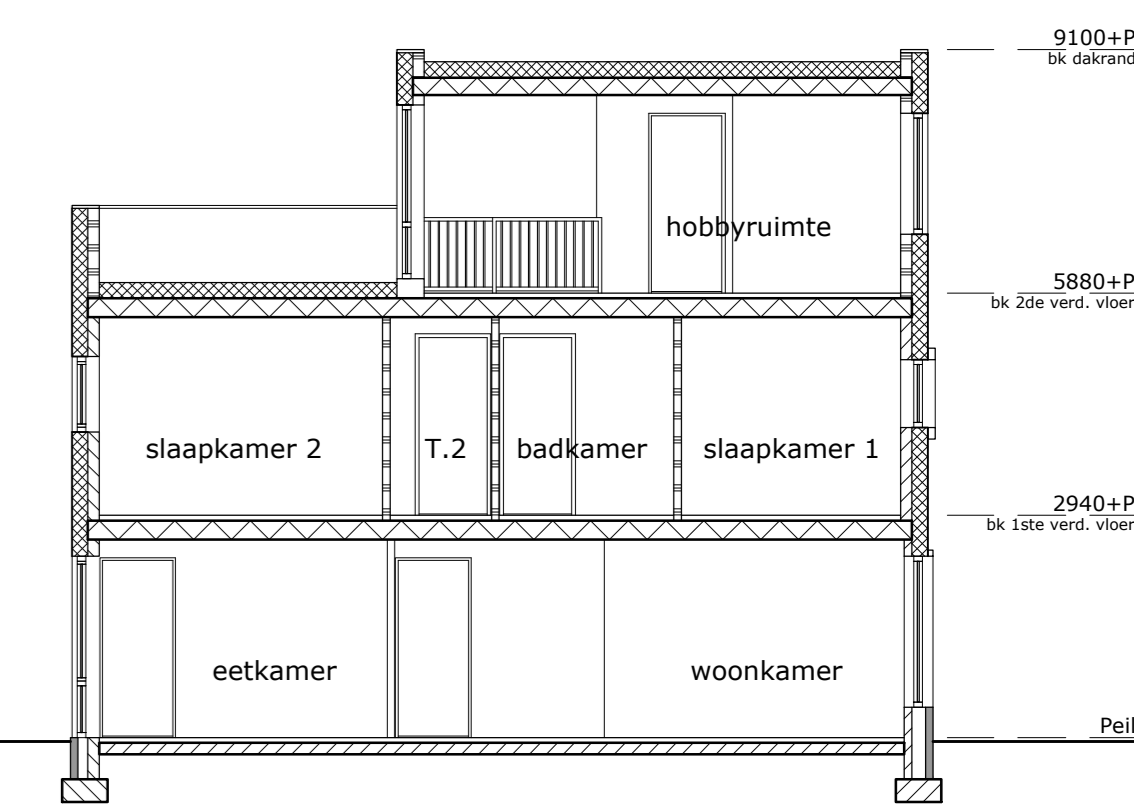
doorsnede schaal 1:100 OPTIE: VERGROTEN HOBBYRUIMTE
