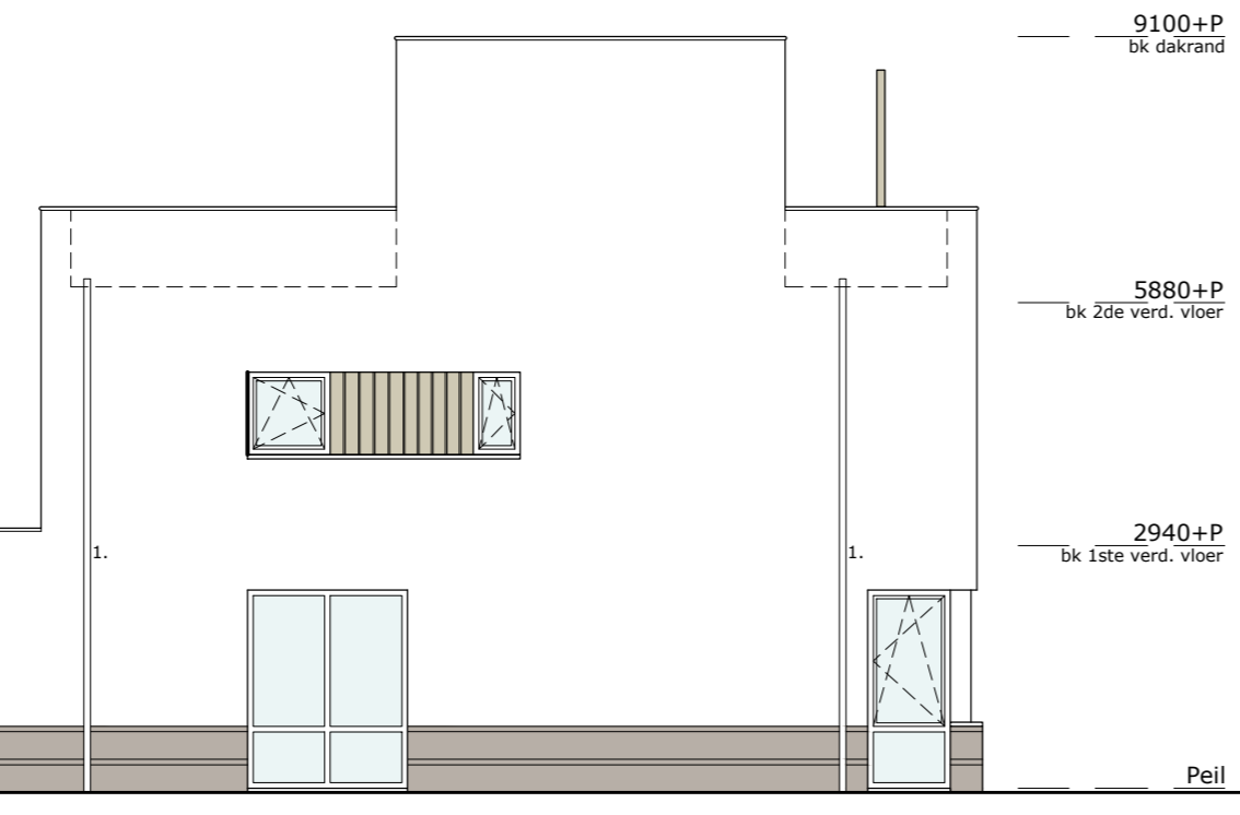
linkerzijgevel schaal 1:100 OPTIE: UITBREIDING 1,20M
