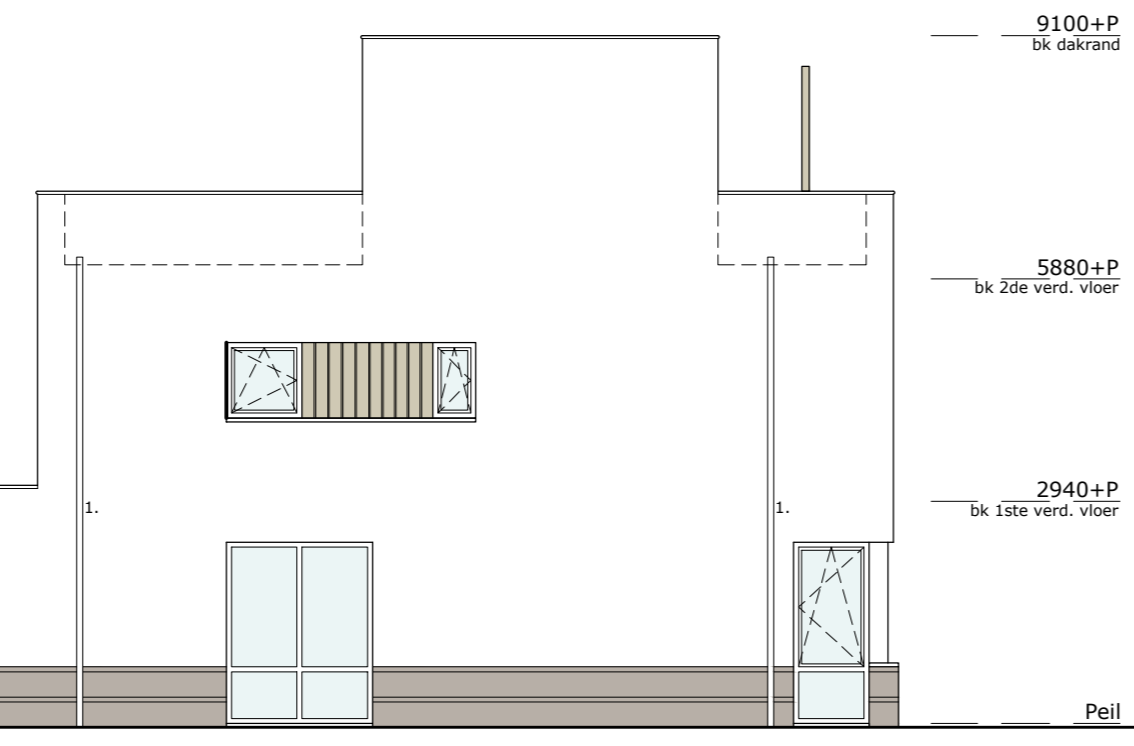
linkerzijgevel schaal 1:100 OPTIE: UITBREIDING 2,40M
