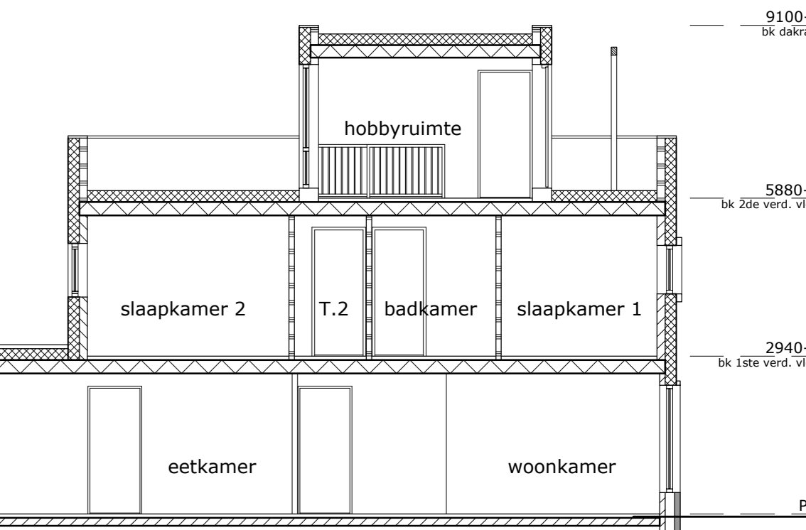
doorsnede schaal 1:100 OPTIE: UITBREIDING 2,40M
