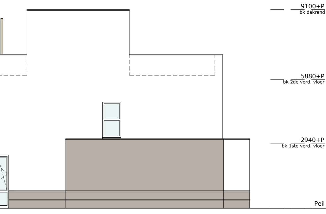
rechterzijgevel schaal 1:100 OPTIE: UITBREIDING 1,20M
