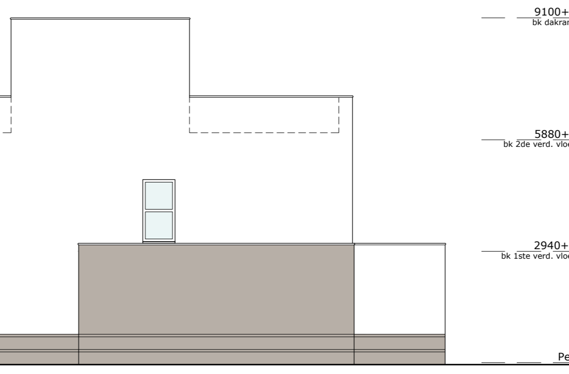
rechterzijgevel schaal 1:100 OPTIE: UITBREIDING 2,40M
