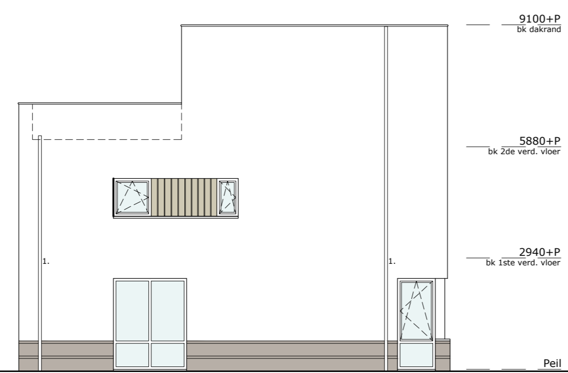
linkerzijgevel schaal 1:100 OPTIE: VERGROTEN HOBBYRUIMTE
