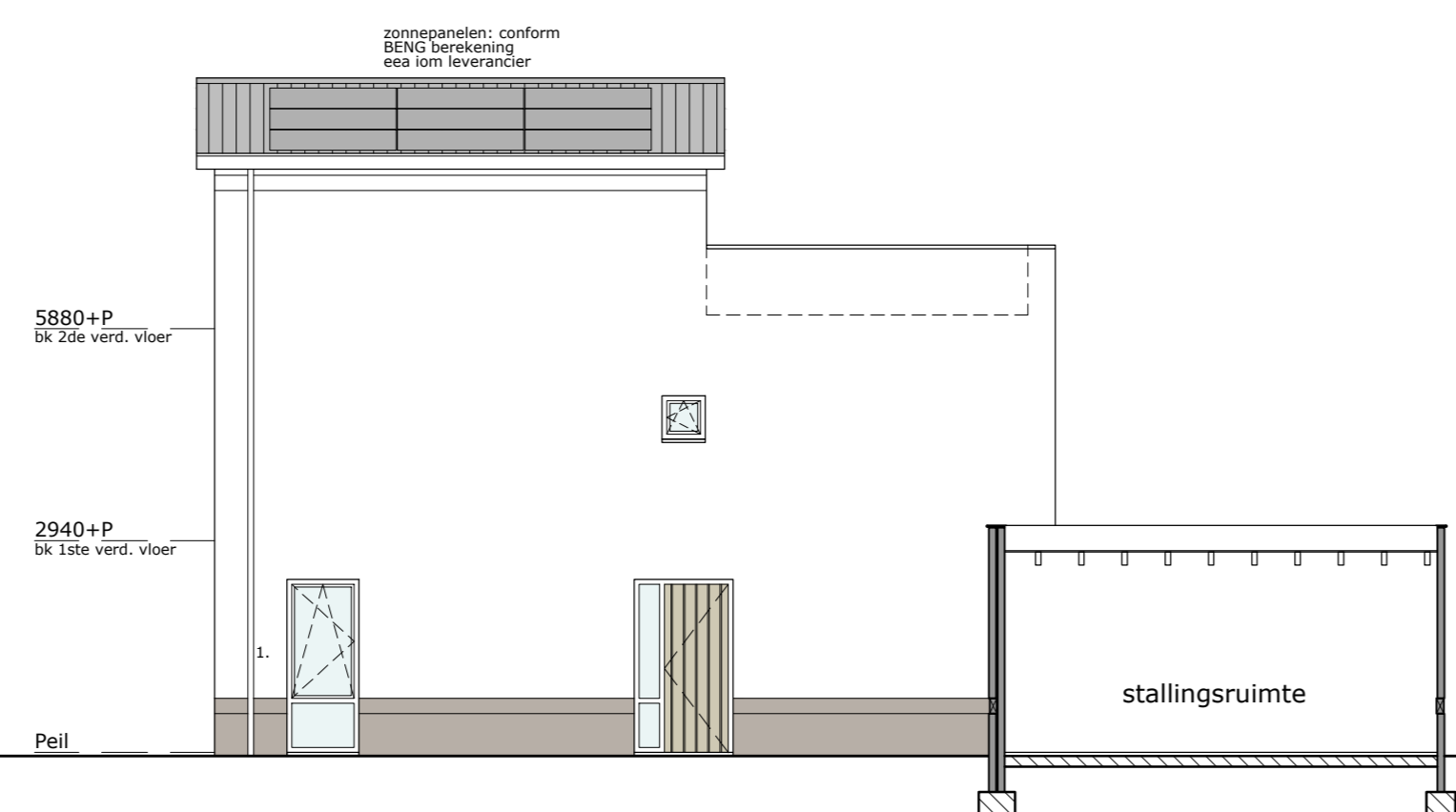
rechterzijgevel schaal 1:100
