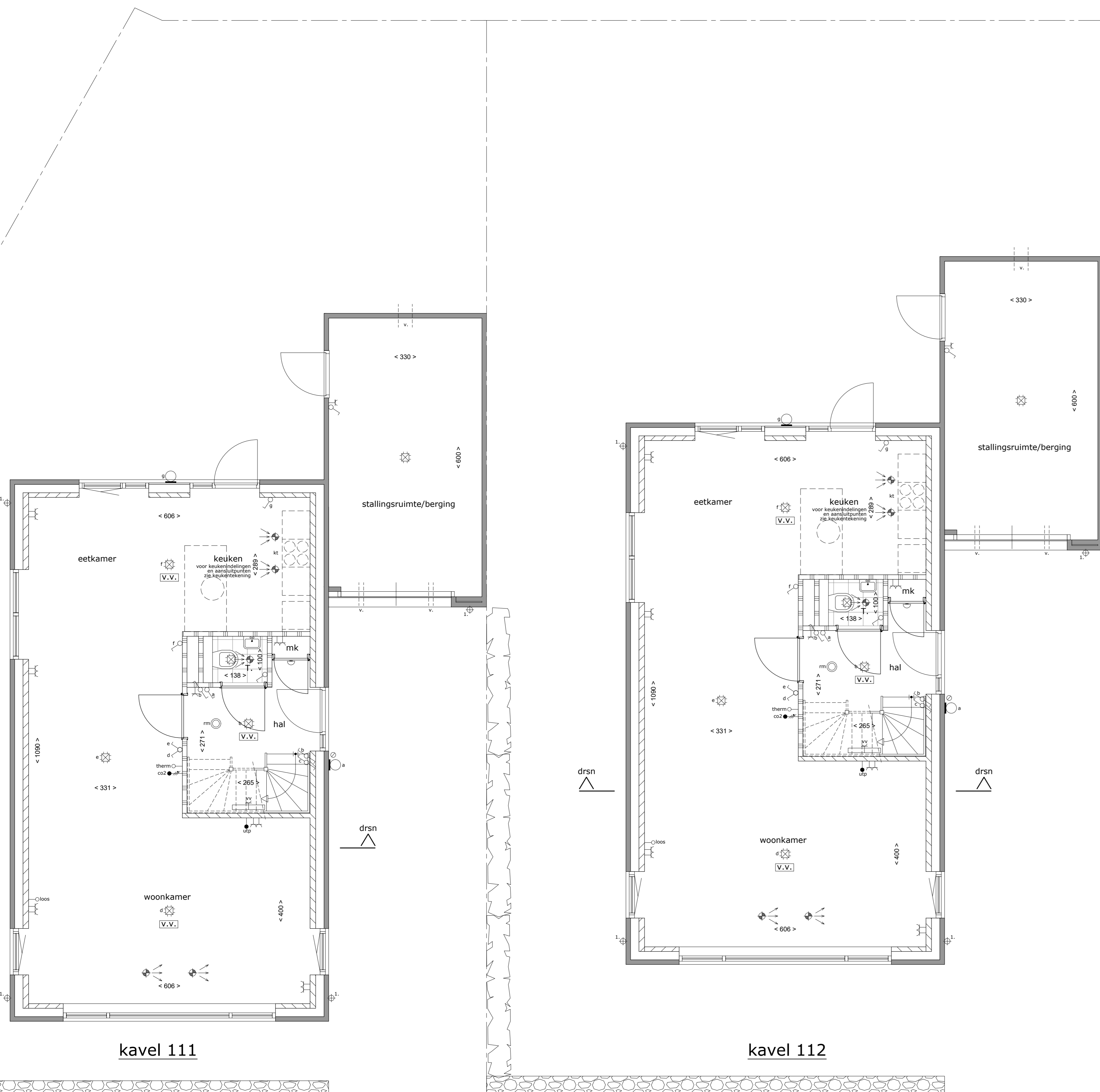
begane grond schaal 1:50
