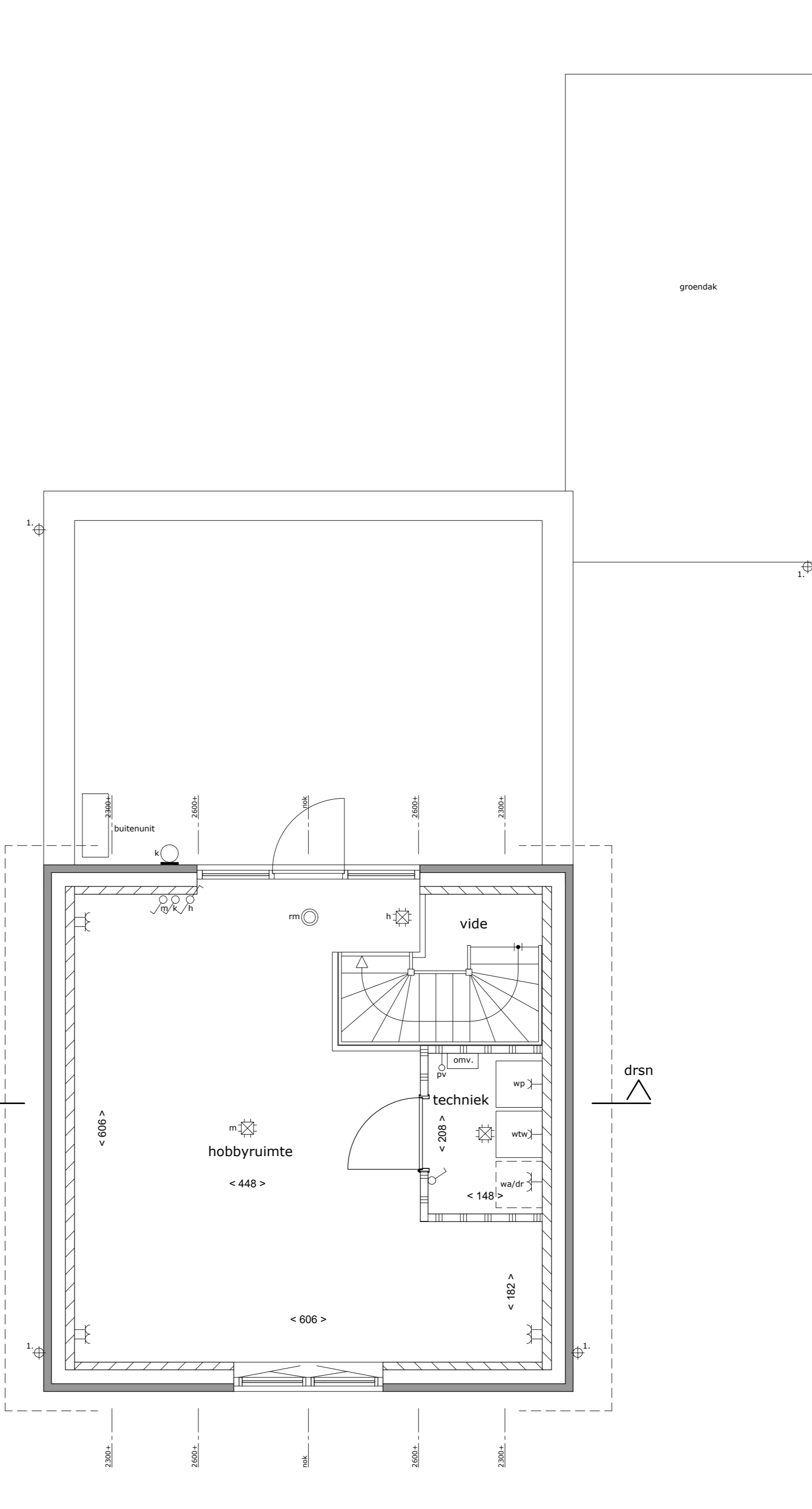
2de verdieping schaal 1:50
