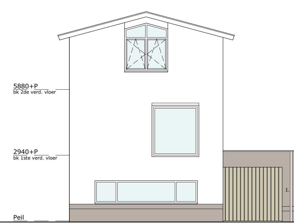
voorgevel schaal 1:100
