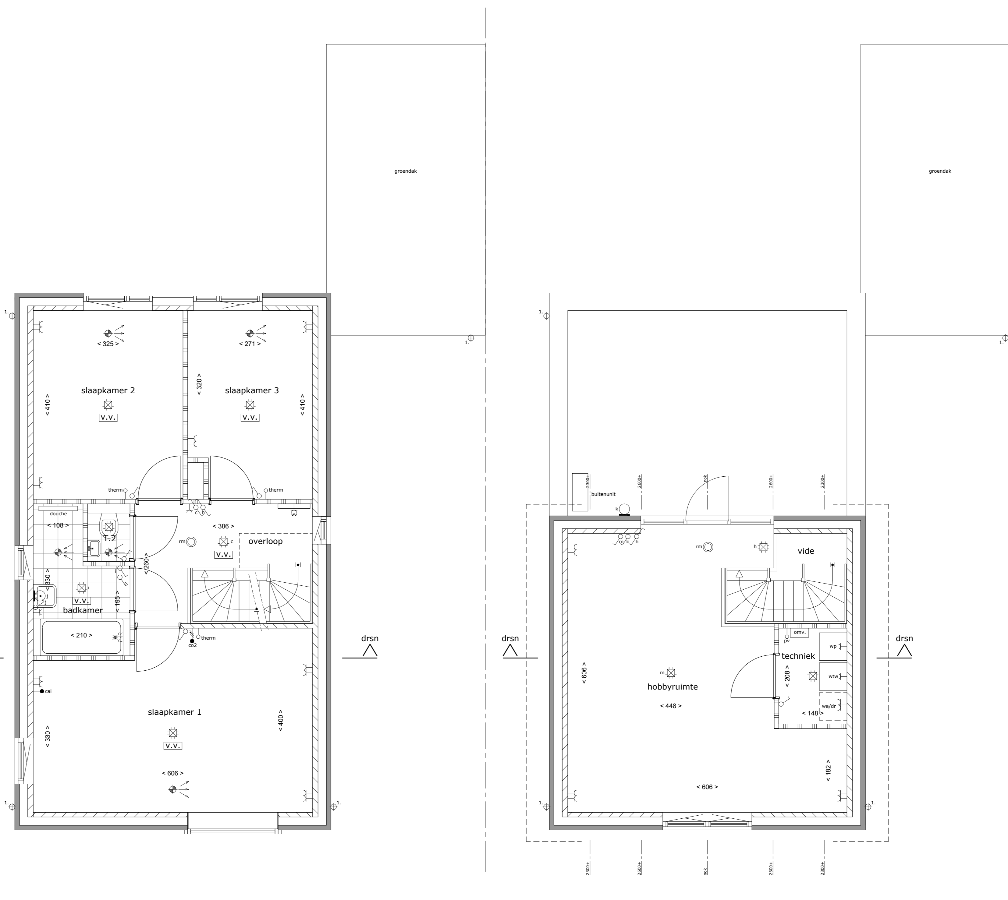
1ste verdieping schaal 1:50
