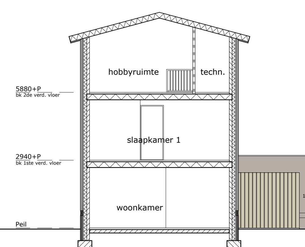
doorsnede schaal 1:100
