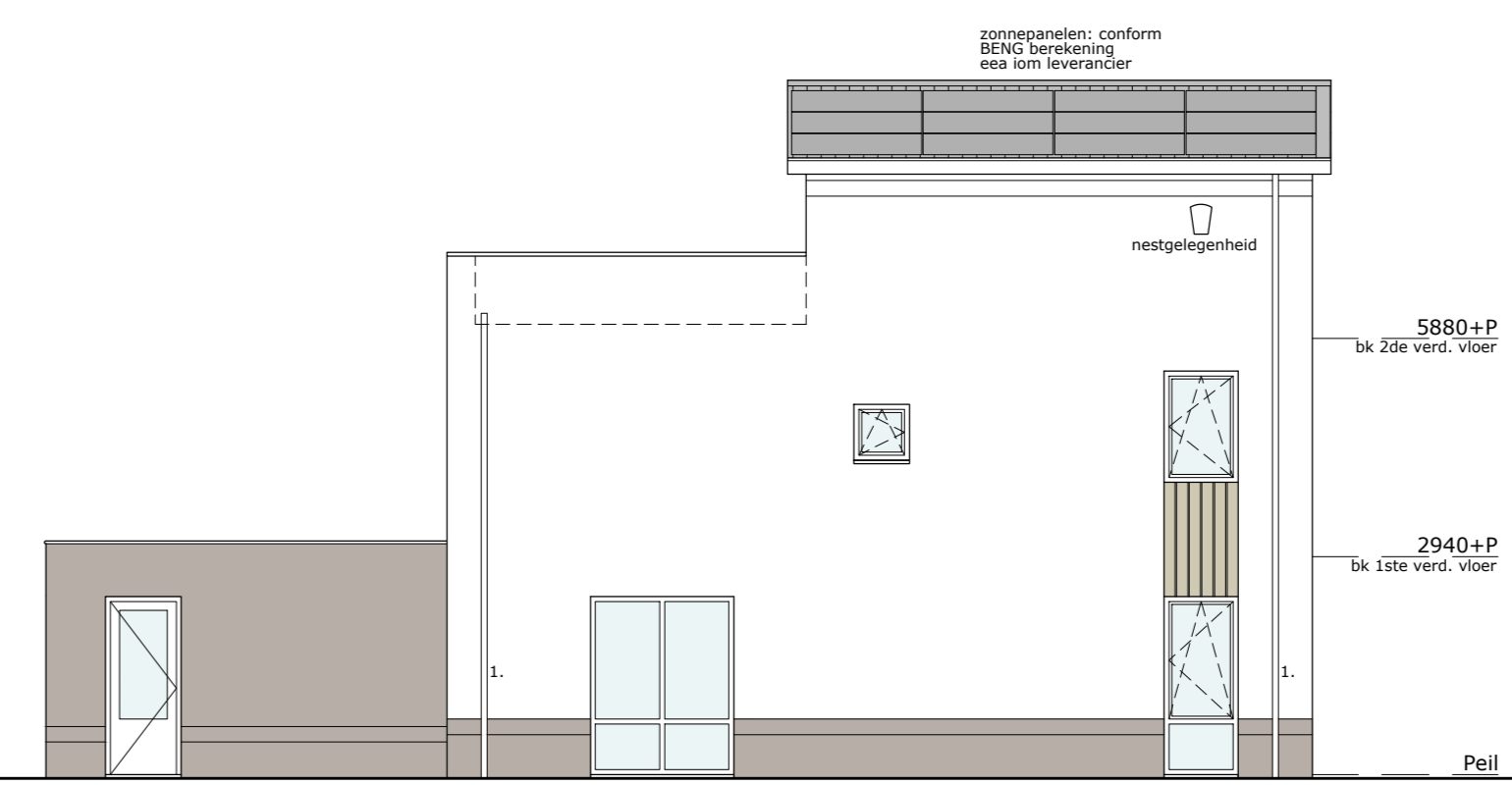
linkerzijgevel schaal 1:100
