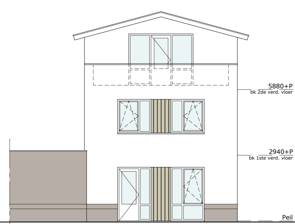
achtergevel schaal 1:100
