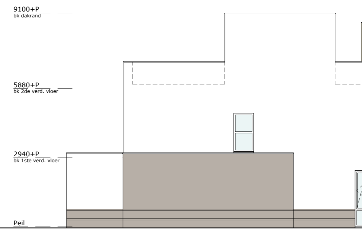
linkerzijgevel schaal 1:100 OPTIE: UITBREIDING 2,40M
