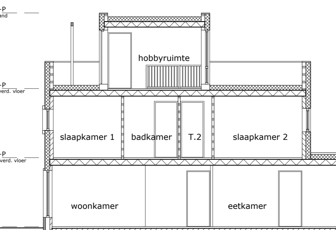
doorsnede schaal 1:100 OPTIE: UITBREIDING 2,40M
