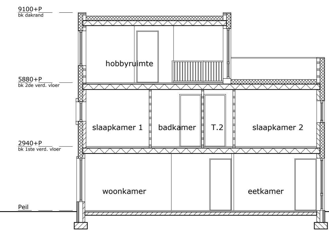
doorsnede schaal 1:100 OPTIE: VERGROTEN HOBBYRUIMTE
