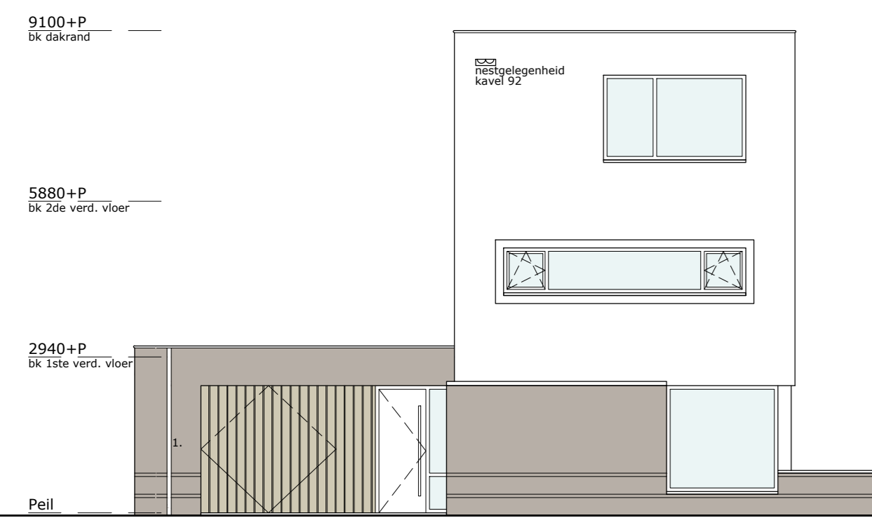
voorgevel schaal 1:100 OPTIE: VERGROTEN HOBBYRUIMTE
