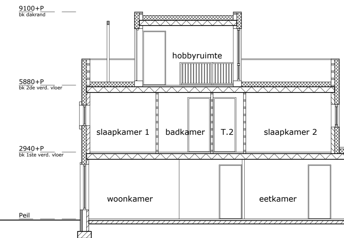
doorsnede schaal 1:100 OPTIE: UITBREIDING 1,20M
