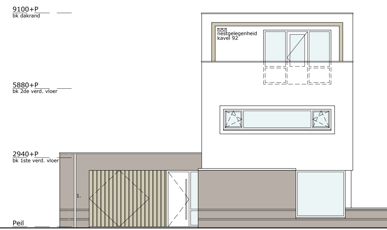
voorgevel schaal 1:100 OPTIE: UITBREIDING 2,40M
