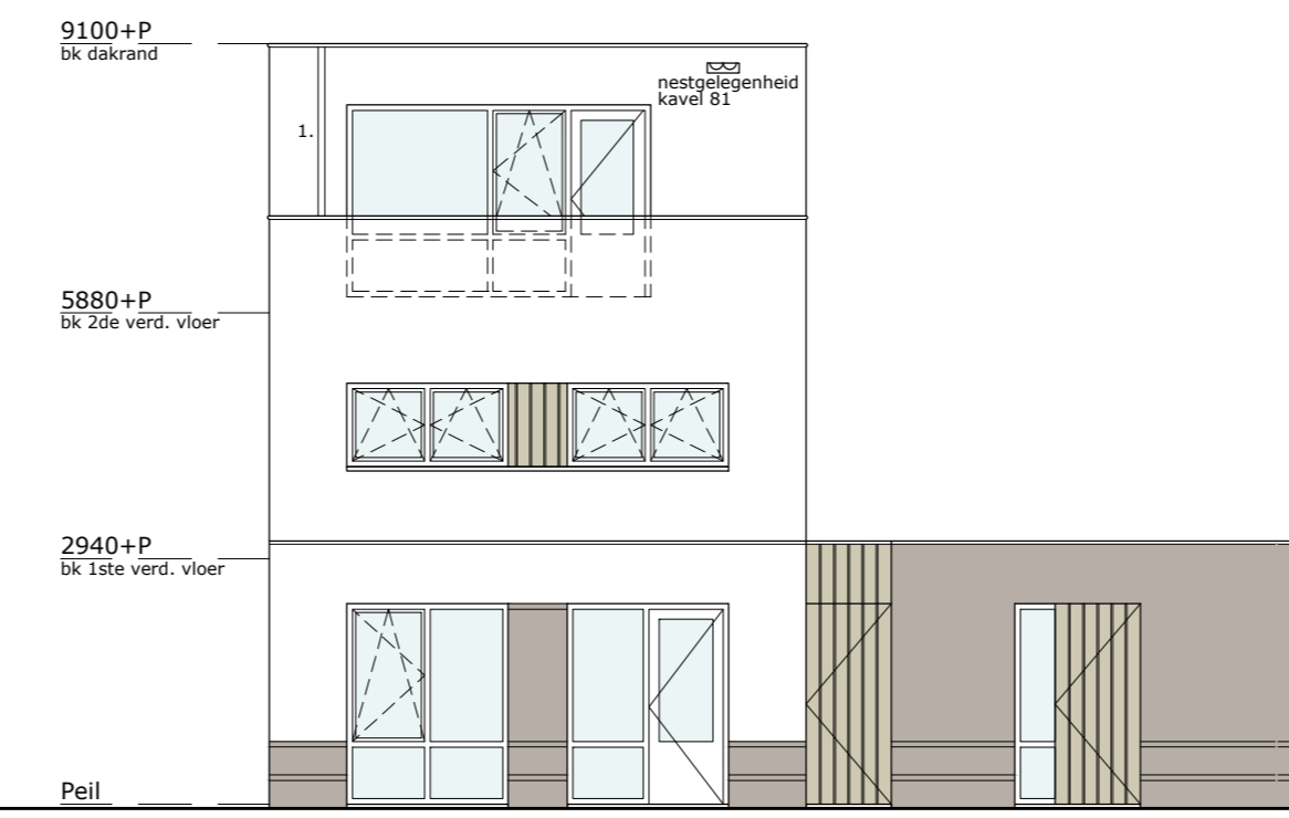
achtergevel schaal 1:100 OPTIE: UITBREIDING 1,20M / 2,40M
