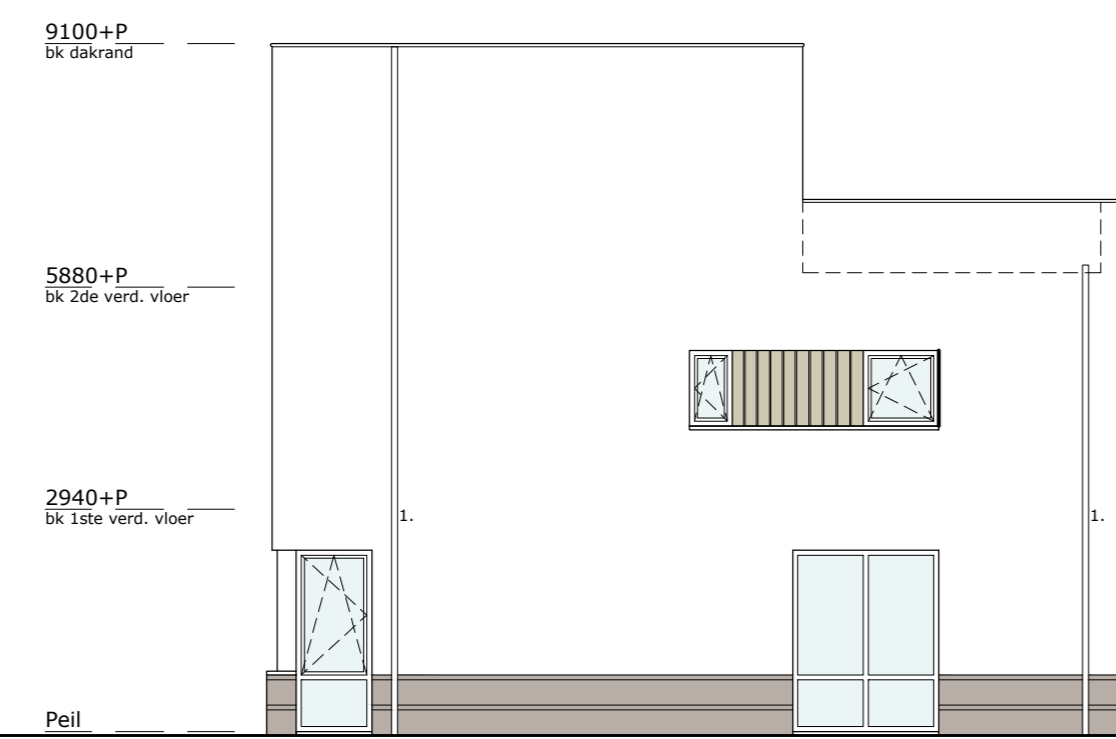
rechterzijgevel schaal 1:100 OPTIE: VERGROTEN HOBBYRUIMTE
