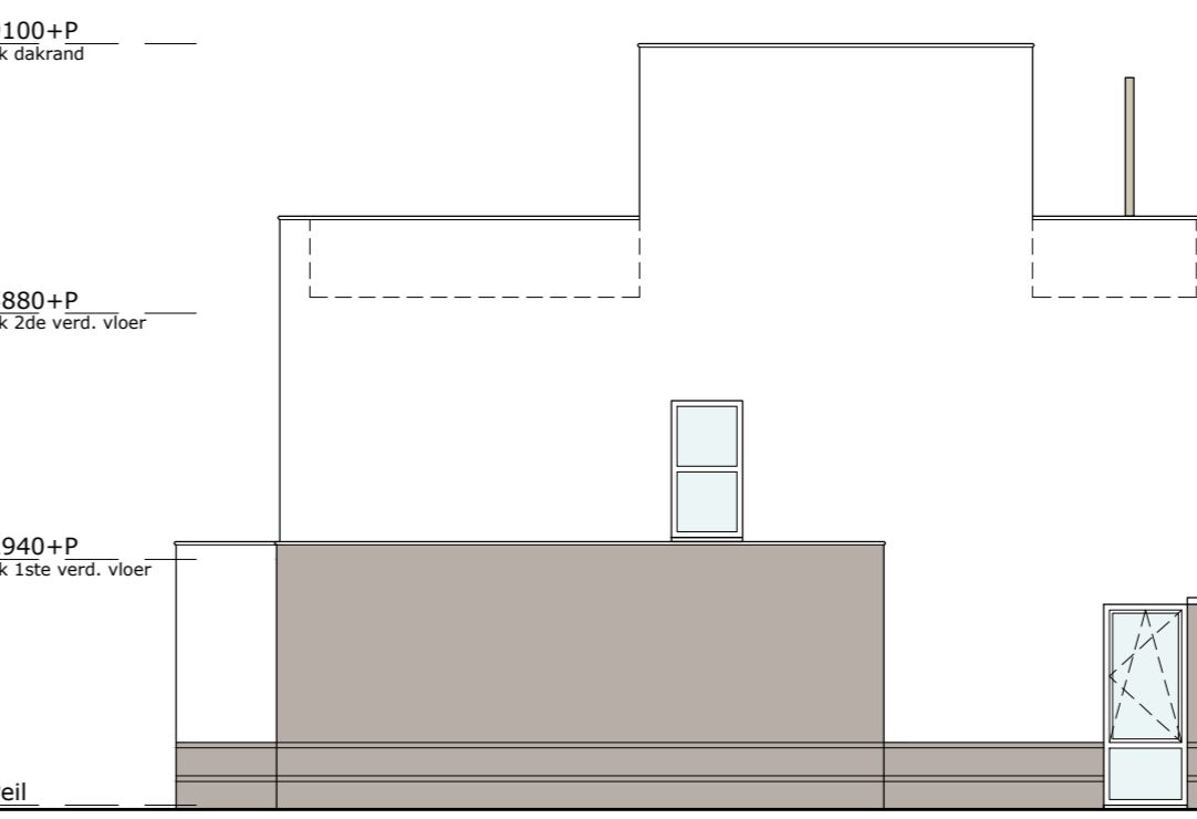
linkerzijgevel schaal 1:100 OPTIE: UITBREIDING 1,20M
