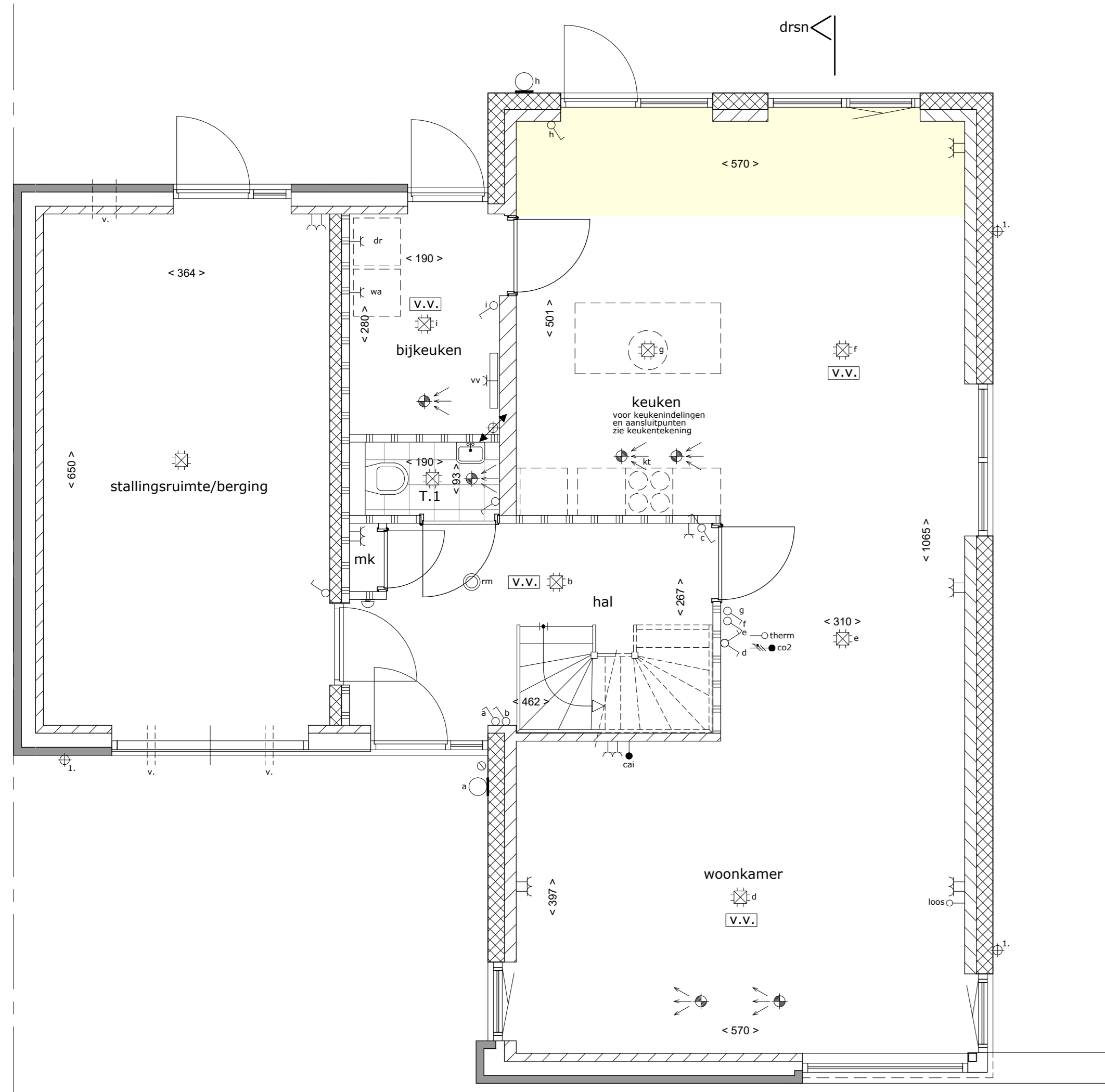
OPTIE: UITBREIDING 1,20M
