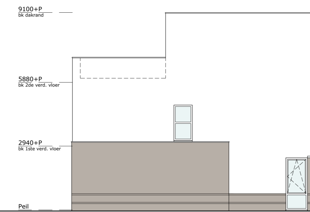
linkerzijgevel schaal 1:100 OPTIE: VERGROTEN HOBBYRUIMTE
