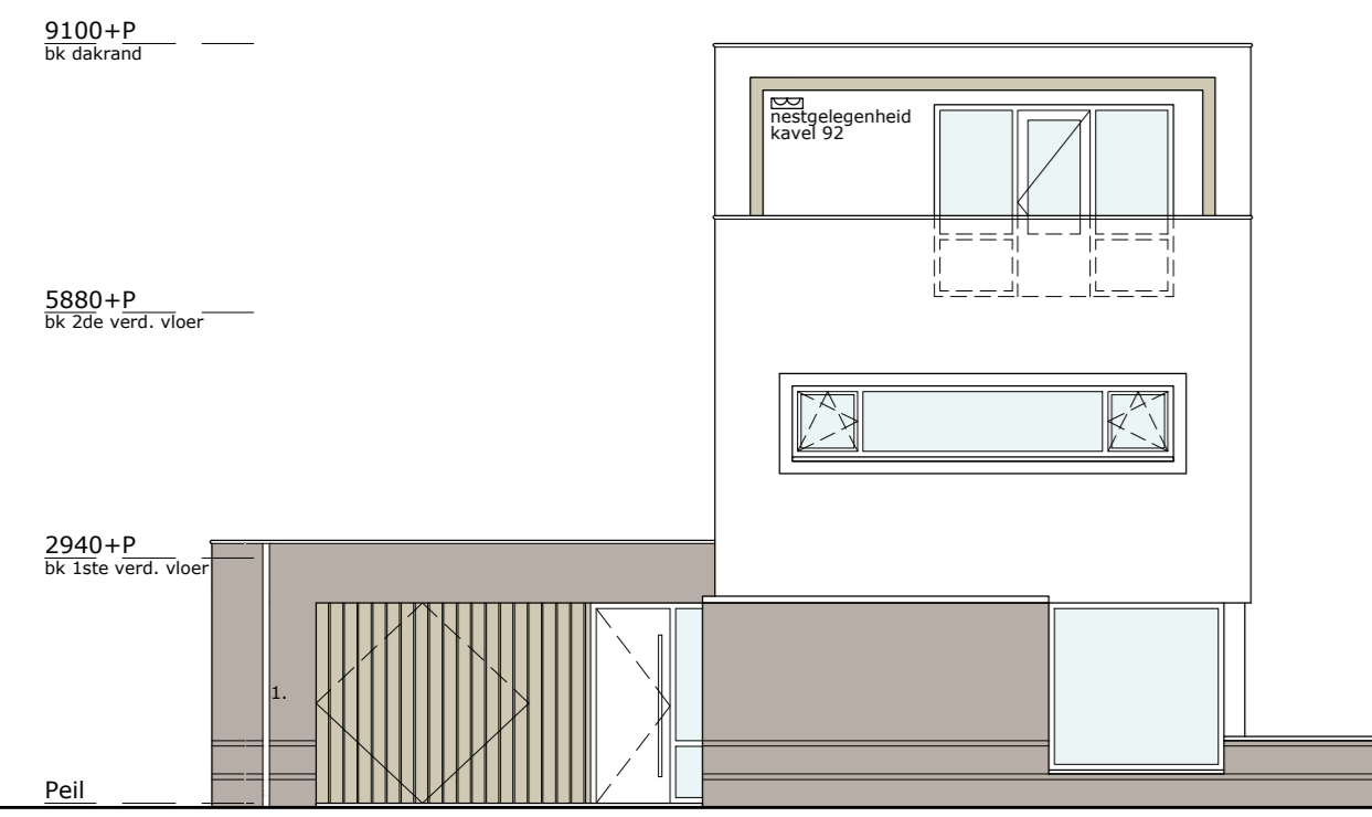
voorgevel schaal 1:100 OPTIE: UITBREIDING 1,20M
