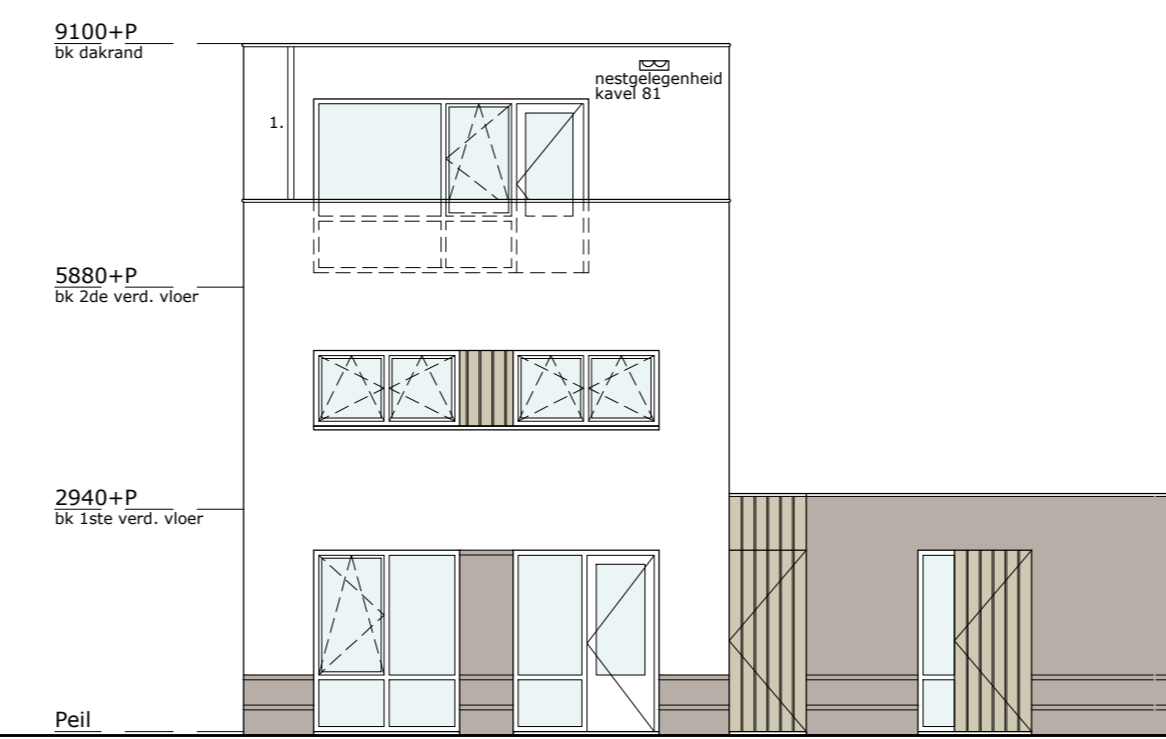
achtergevel schaal 1:100 OPTIE: VERGROTEN HOBBYRUIMTE
