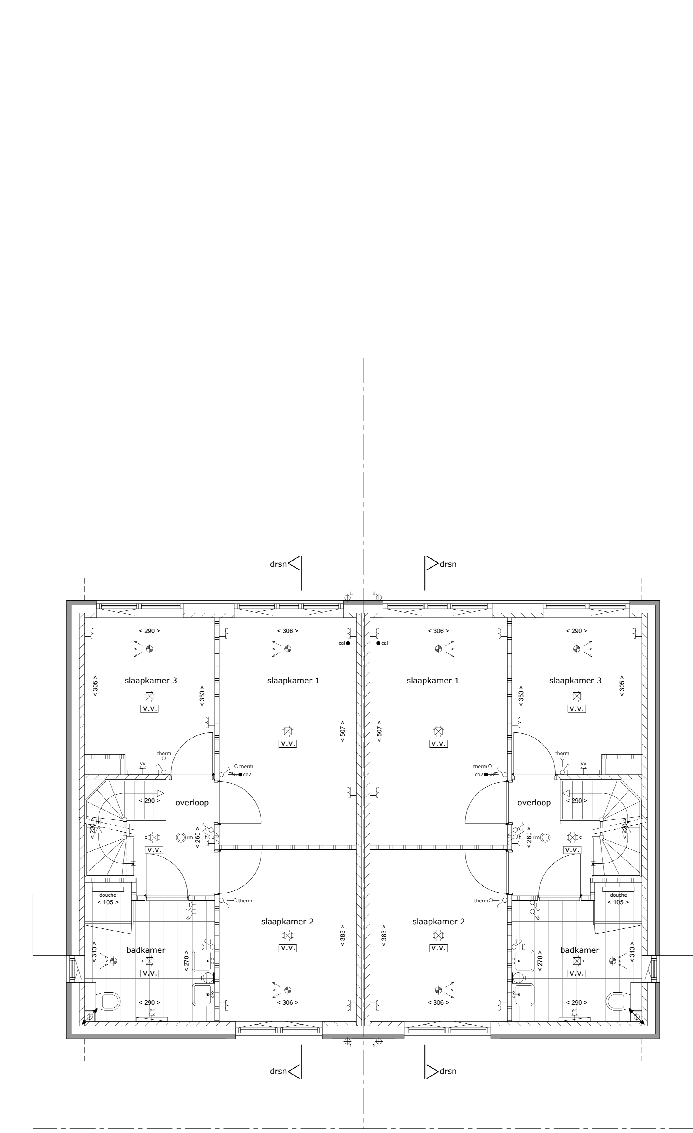
kavel 107 kavel 108 1ste verdieping schaal 1:50
