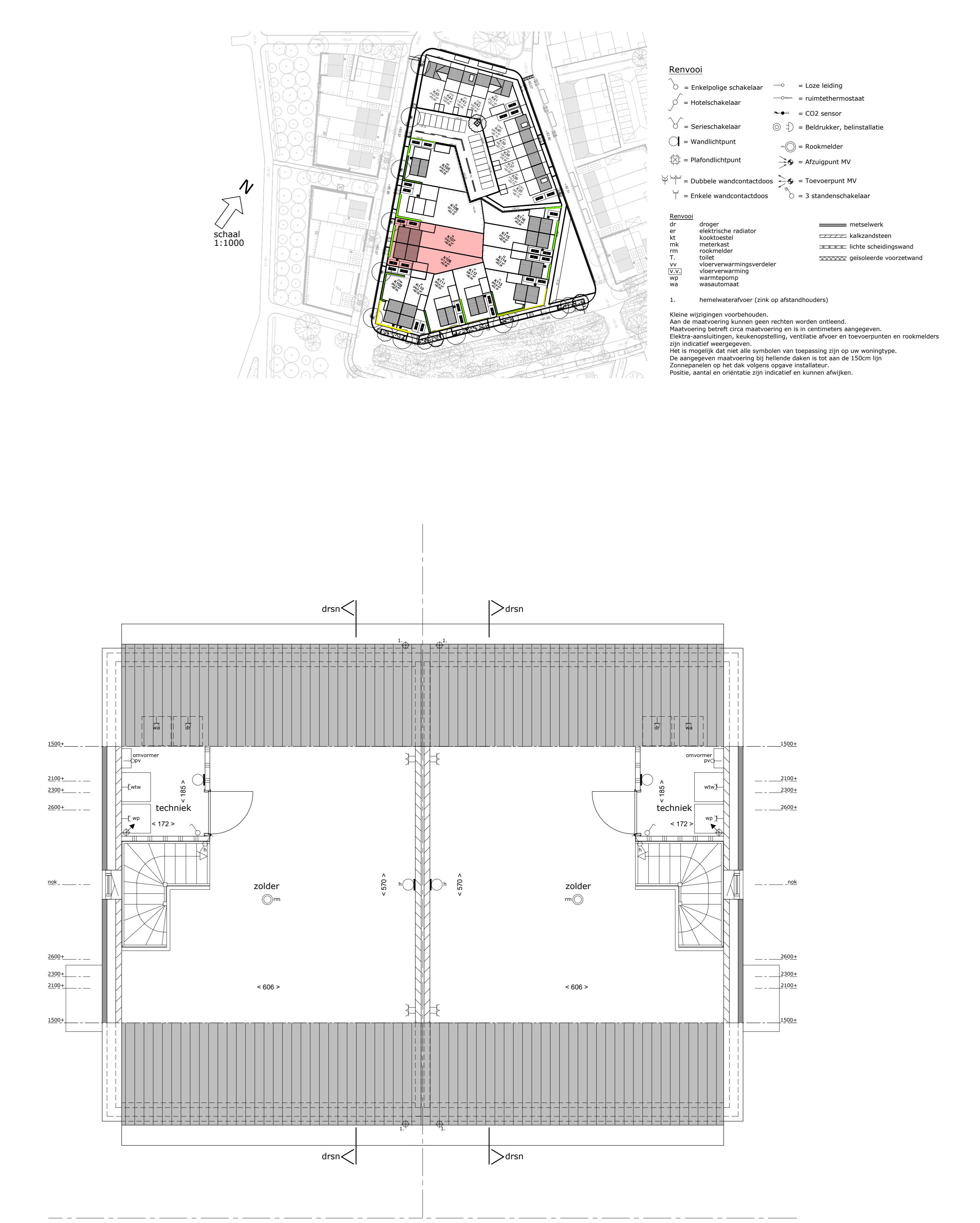
kavel 107 kavel 108 2de verdieping schaal 1:50
