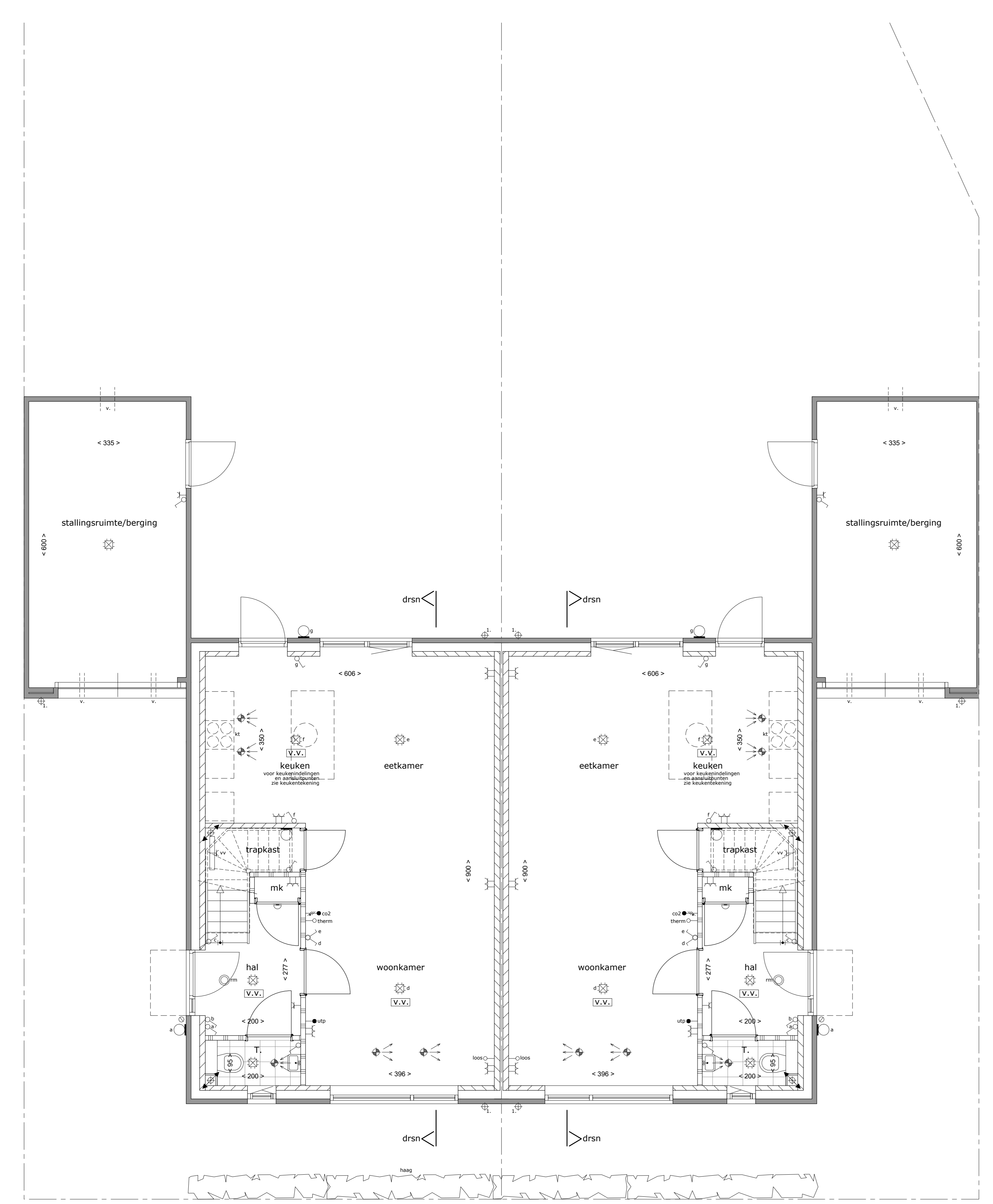
kavel 107 kavel 108 begane grond schaal 1:50
