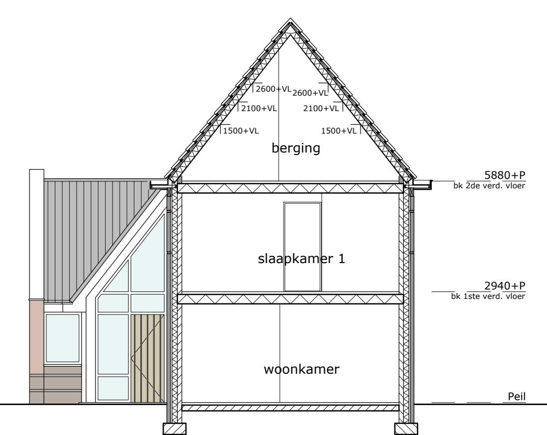
doorsnede schaal 1:100
