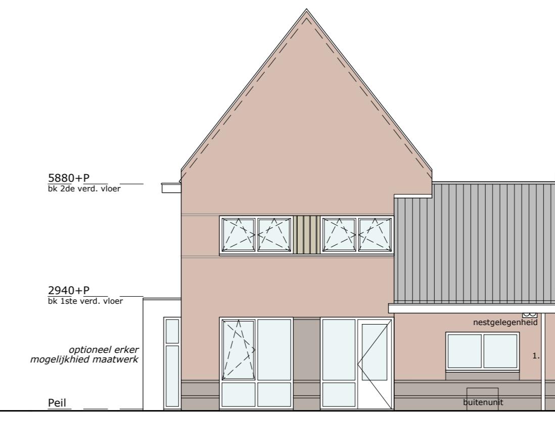
achtergevel schaal 1:100
