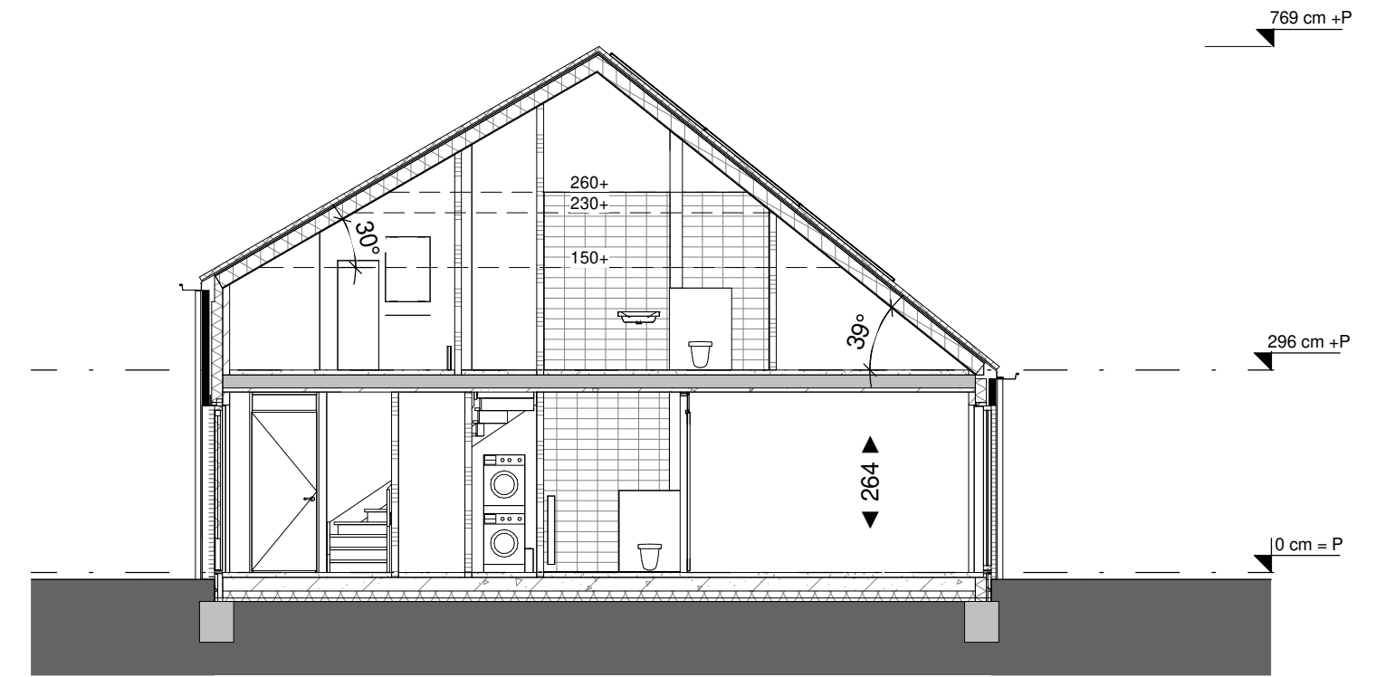
Doorsnede A
