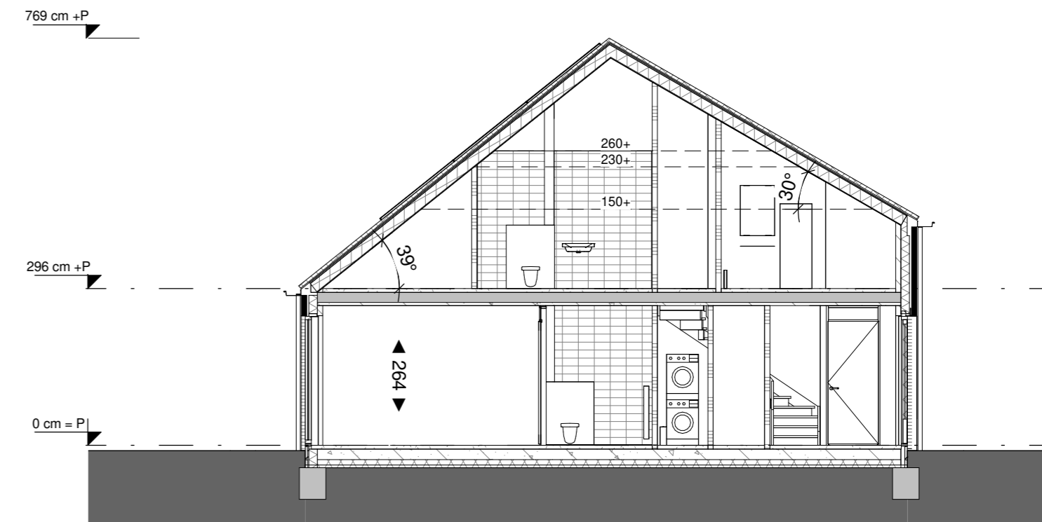
Doorsnede A
