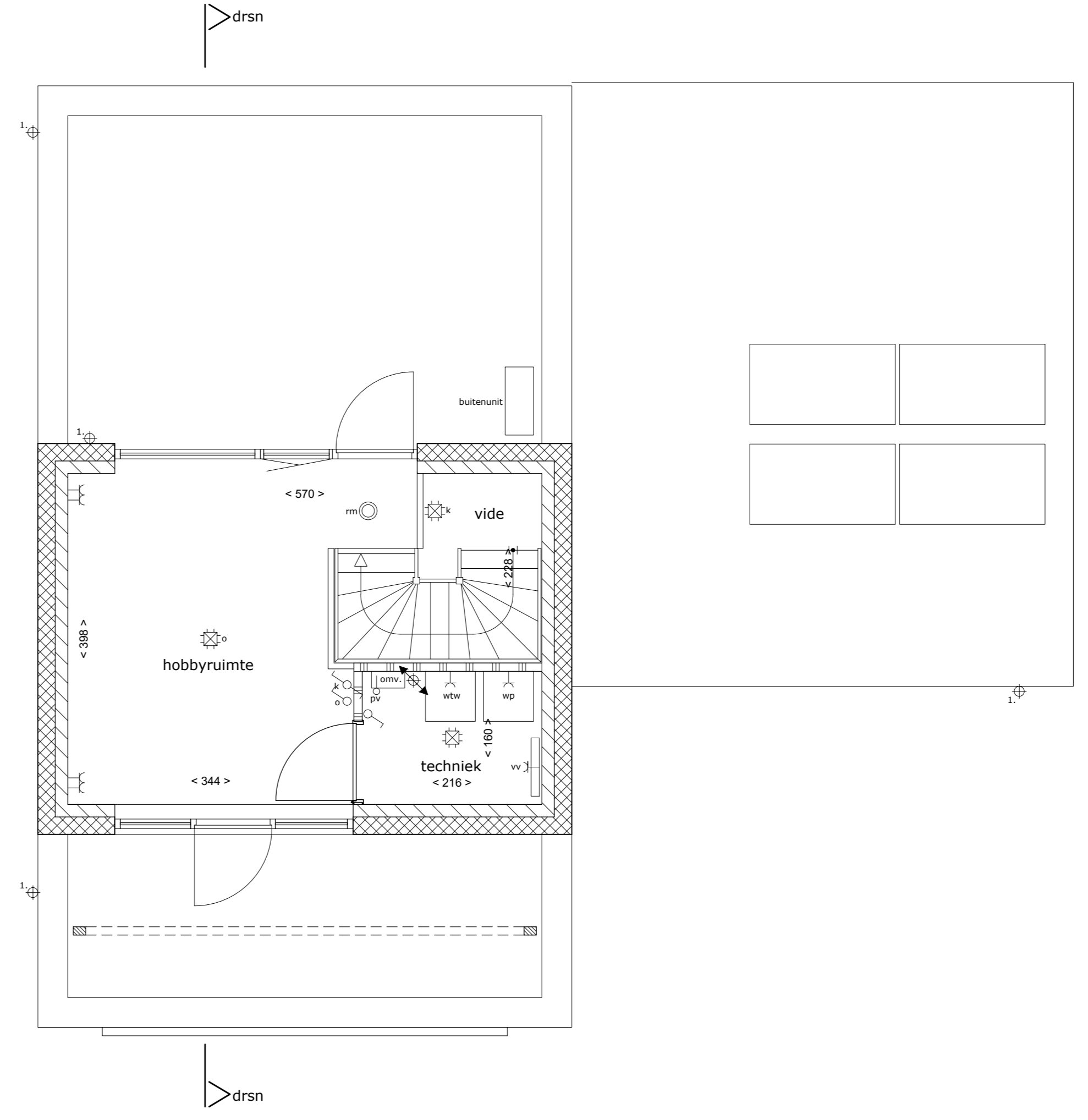
2de verdieping schaal 1:50
