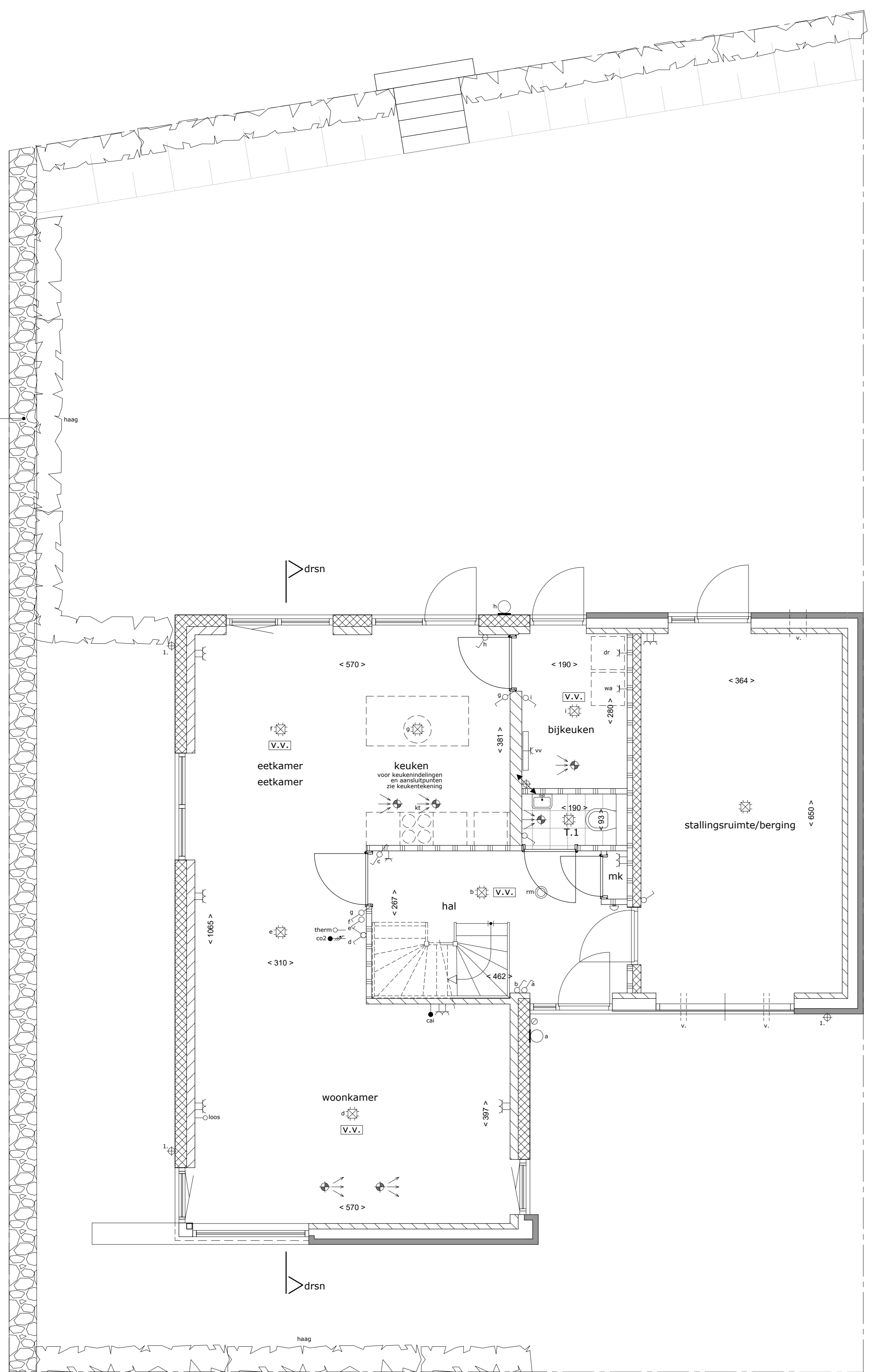
begane grond schaal 1:50
